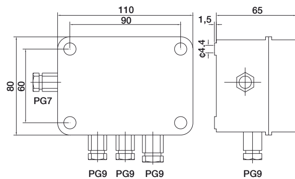
Massbild Aufbaugehäuse ESAS 25
